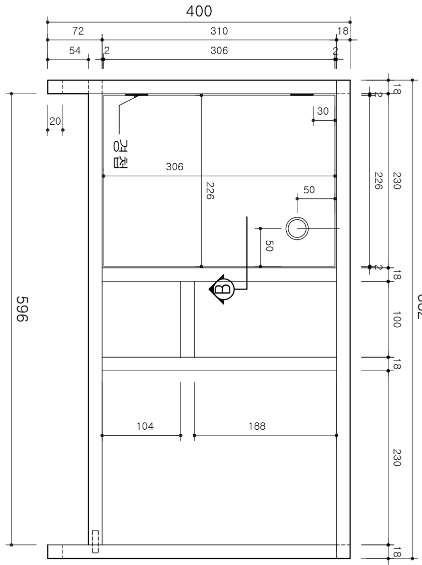
정면도 SCALE 1:5
