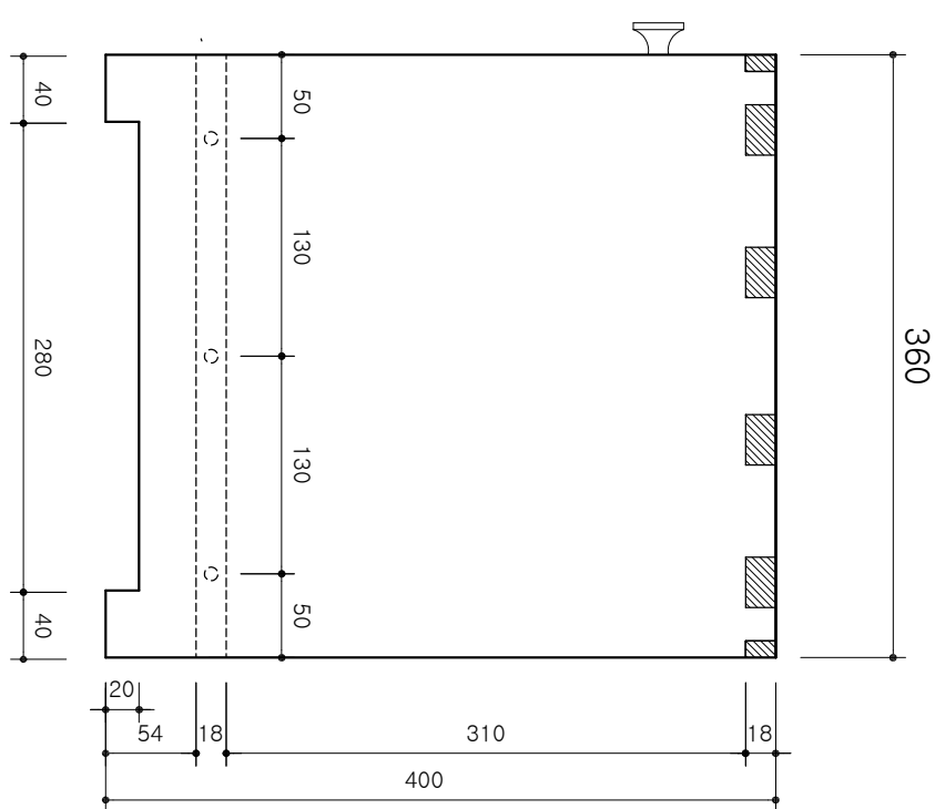
우측면도 SCALE 1:5
